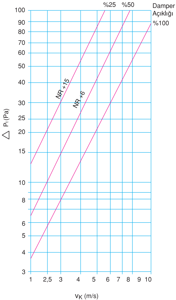
BASINÇ KAYBI DİYAGRAMI
